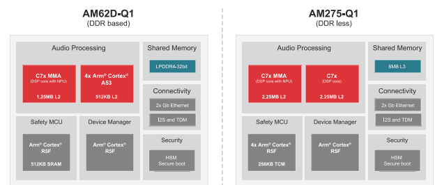
그림 6. AM2754-Q1 및 AM62D-Q1에서 볼 수 있는 높은 수준의 통합.
