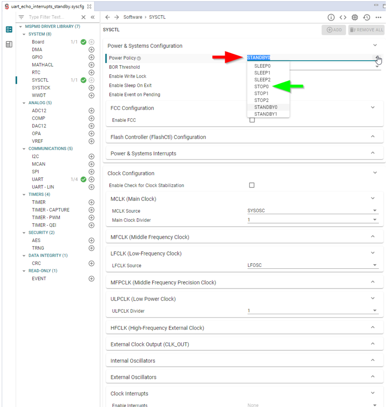
그림 2-7. 전원 모드 구성
