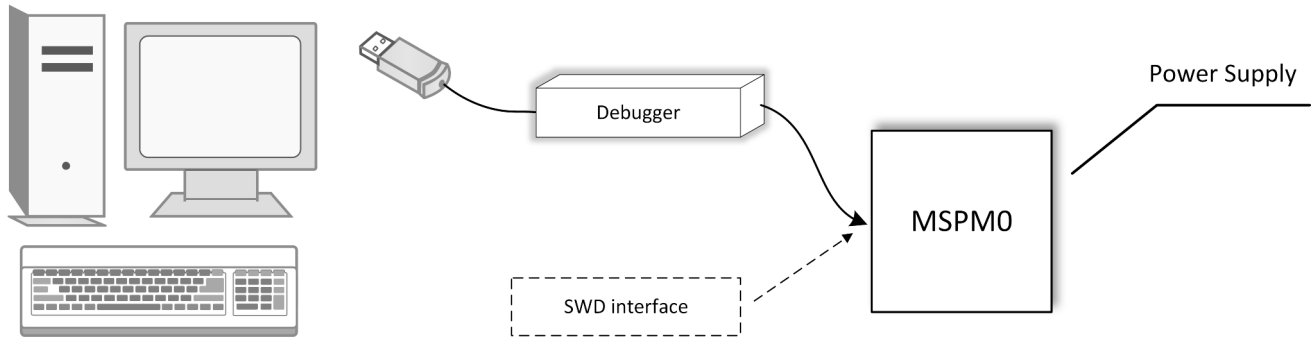
그림 2-3. MSPM0 디버깅
