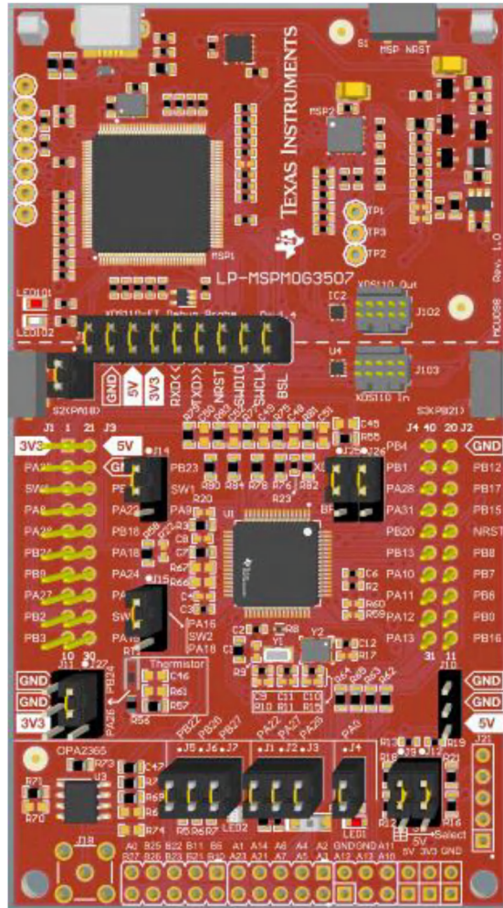
그림 2-2. LP-MSPM0G3507 LaunchPad 개발 키트
