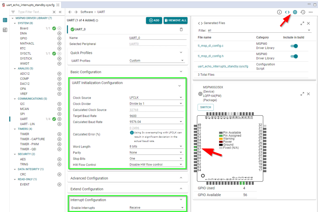
그림 2-8. UART 구성
