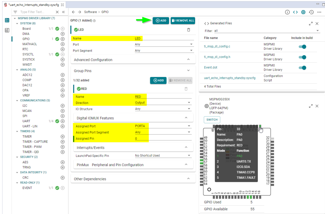
그림 2-9. GPIO 구성
