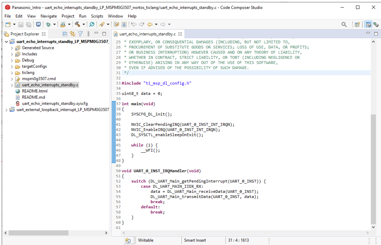
그림 2-6. uart_echo_interrupts_standby 예제
